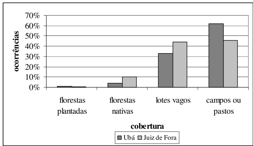
Figura 4 – Ocorrências de incêndios de acordo com o material combustível
