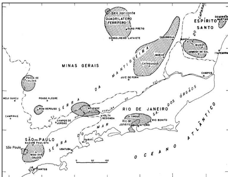
Figura 3. Província bauxitífera do sudeste, principais depósitos conhecidos. (Kotschoubey, 1988: 608).
