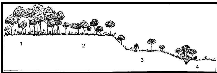
FIGURA 4 – Perfil de fitofisionomias do bioma Cerrado. 1- Cerrado Denso 2- Cerrado Típico 3- Cerrado Ralo 4- Campos. Fonte: RADAMBRASIL (1984).
