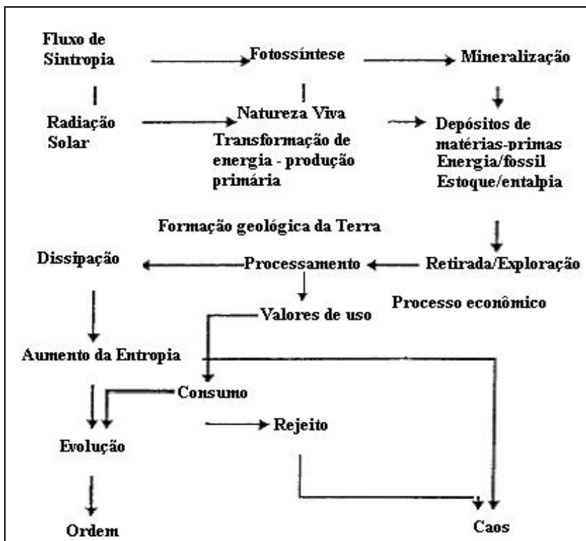
Figura 1. Fluxo de sintropia e aumento de entropia (Altvater, 1995:50)
