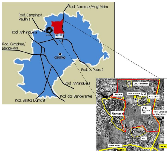
Figura 1: Localização do CIATEC II no Município de Campinas (no destaque)
