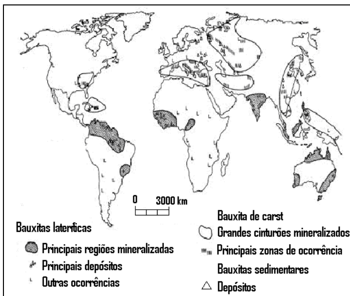
Figura 2. Distribuição mundial dos depósitos de bauxita. (Kotschoubey (1988, p. 605)
