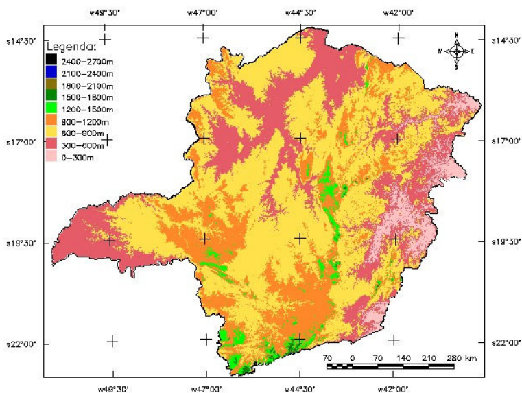
FIGURA 2 – Cotas altimétricas obtidas através dos dados SRTM para o Estado de Minas Gerais.
